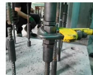
垂直度调整
