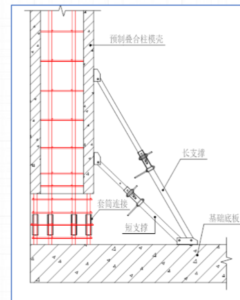
斜支撑示意 (如有)
