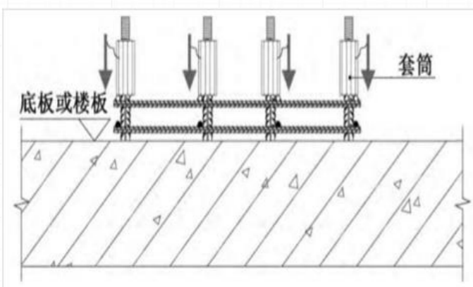
箍筋预放
